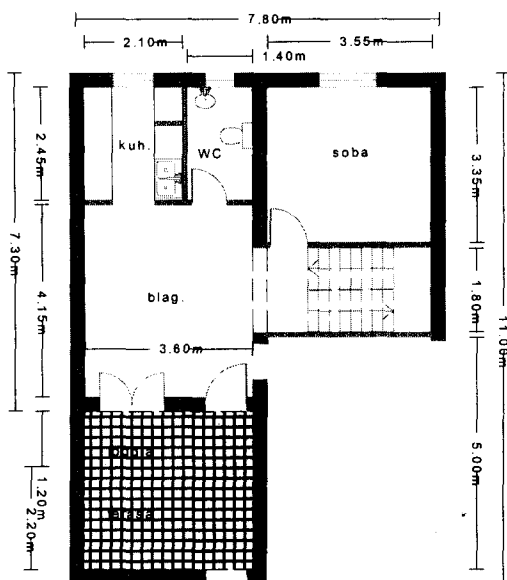
tlocrt prizemlja
