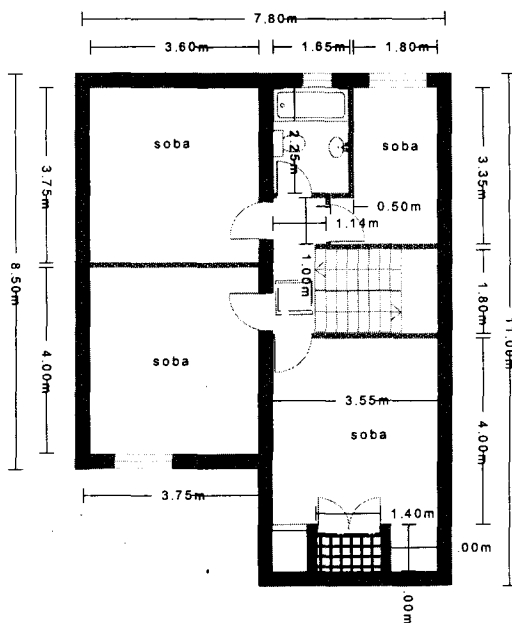
tlocrt visokog potkrovlja
